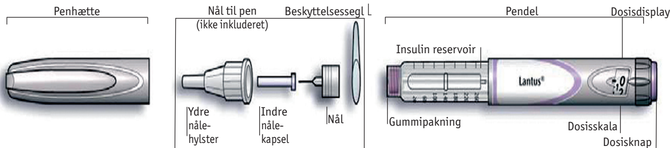
Schematisk diagram af pennen
