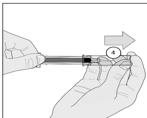
Figur 3. Injektionssprøjte med et manuelt sikkerhedssystem, hvor en sikkerhedsmanchet bliver trukket hen over nålen efter brug .
